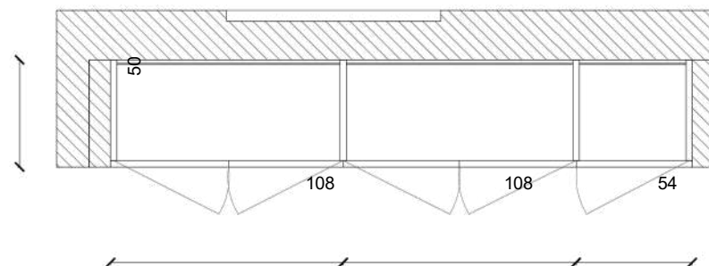
Pianta
