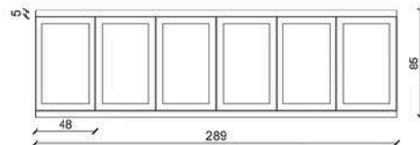
Prospetto chiuso
